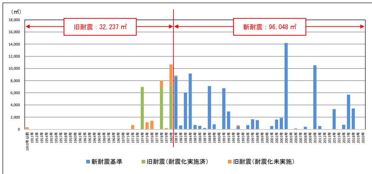
図 3-1-5 建築年別耐震化状況
