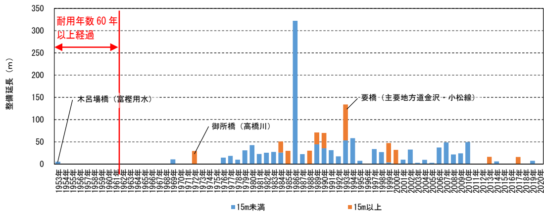
図 3-2-3 橋梁の年度別整備状況
