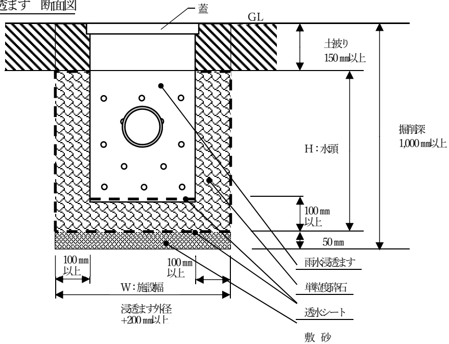
雨水浸透ます 断面図
