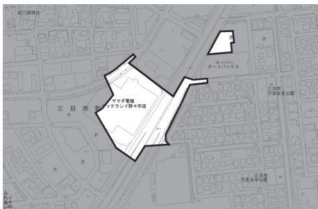
上林の一部
